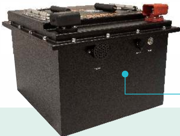
Общий вид литиевого аккумулятора. Привычные терминалы подключения (крепление болт М8)
